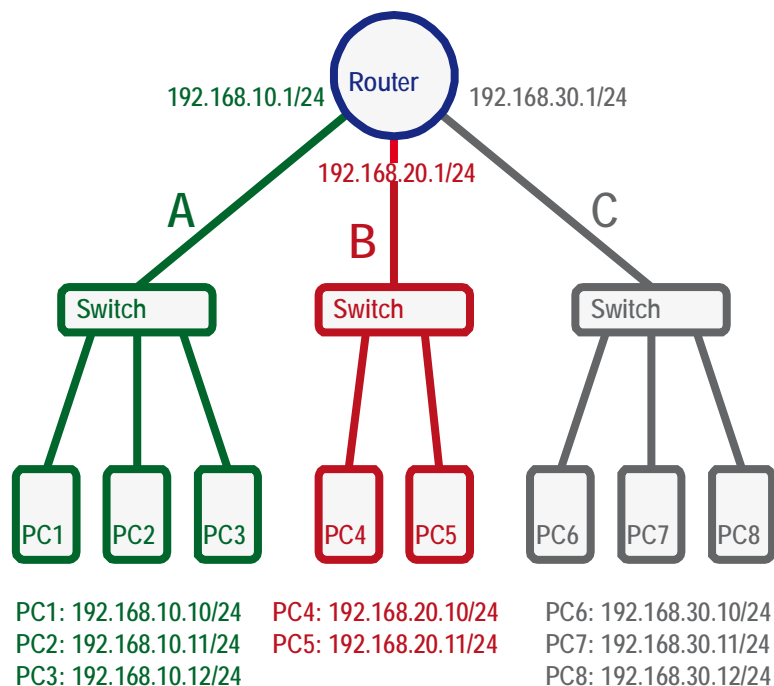
Abbildung 4: Die Grafik zeigt drei getrennte Netze, die über einen Router verbunden sind. Bei den PCs und bei den Router-Schnittstellen sind die IP-Adressen und Subnetzmasken angegeben (/24 ist dabei eine gebräuchliche Abkürzung für die Subnetzmaske 255.255.255.0).
