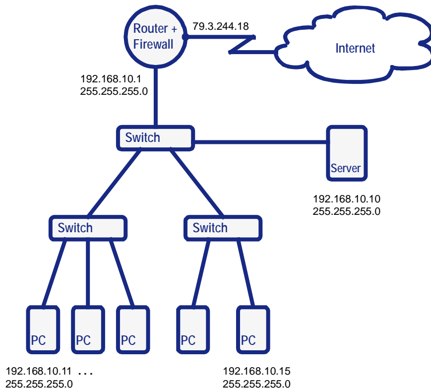
Abbildung 7: Öffentliche und private IP-Adressen; nur die externe Schnittstelle des Routers hat eine öffentliche IP-Adresse und ist aus dem Internet erreichbar.
