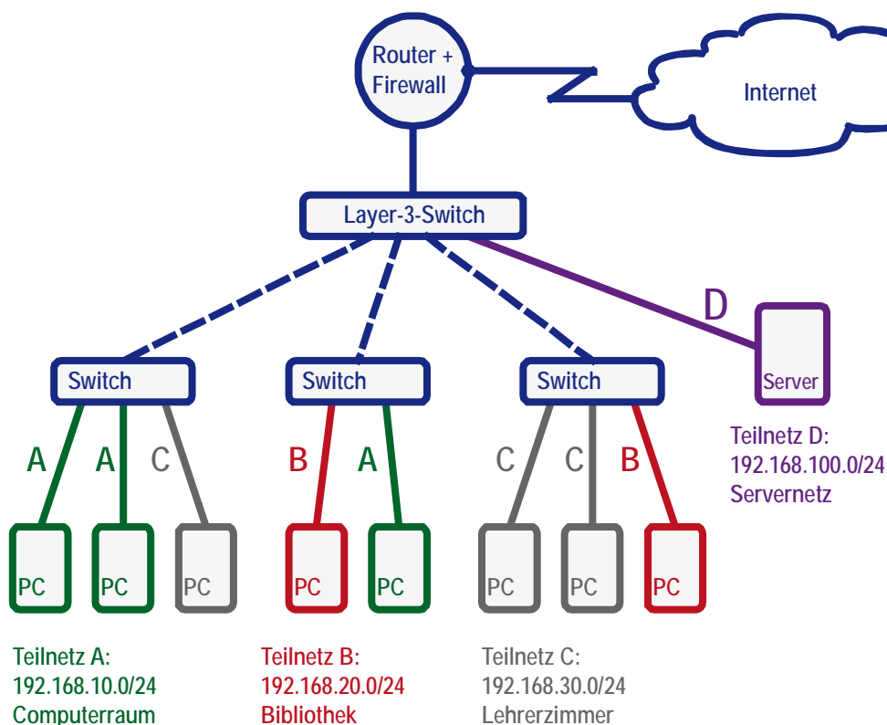
Abbildung 6: In der Grafik ist das lokale Netz in VLANs (A, B, C, D) unterteilt. Die unterbrochen gezeichneten Linien sind Trunk-Leitungen.
