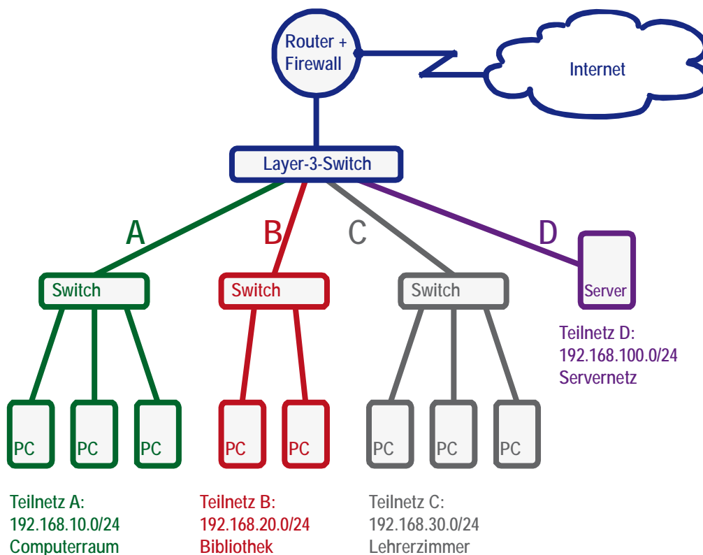
Abbildung 5: Beispielkonfiguration einer größeren Schule mit mehreren getrennten Teilnetzen und eigenem Servernetz. Am Layer-3-Switch wird das lokale Netz in die Teilnetze A, B, C, D getrennt. Der Layer-3-Switch regelt, welche Teilnetze aufeinander zugreifen dürfen. (In der Skizze sind die Netzwerkadressen der Teilnetze angegeben, nicht die IP-Adressen der einzelnen Computer.)
